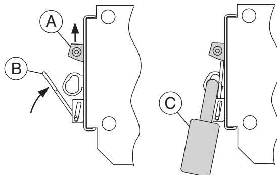
Figure / Figura / Figure 6 : ON Position Locking / Posición de bloqueo en cerrado (I/ON) / Verrouillage en position de marche (I)
