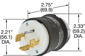
HBL7411C
