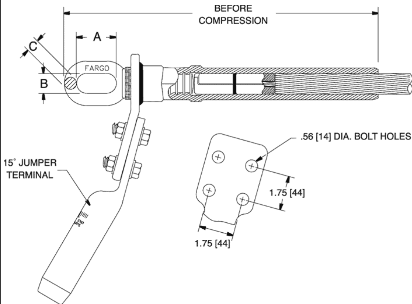
Dimensions
