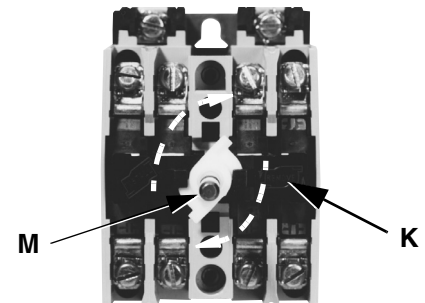
FIG. 2 : T-bar Actuator / Accionador de barra en T / Actionneur à barre en T
