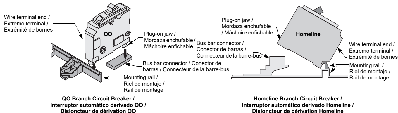
Figure / Figura / Figure 3 : QO or Homeline Branch Circuit Breakers / Interruptores automáticos derivados QO o Homeline / Disjoncteurs de dérivation QO ou Homeline
