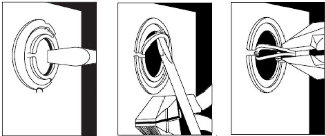
Removing Knockouts / Extracción de los discos desprendibles / Retrait des débouchures
