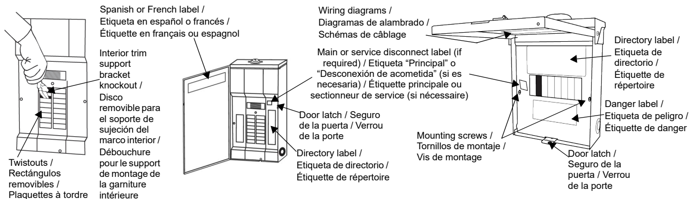
Figure / Figura / Figure 5 : Label Application / Cómo colocar las etiquetas / Application des étiquettes
