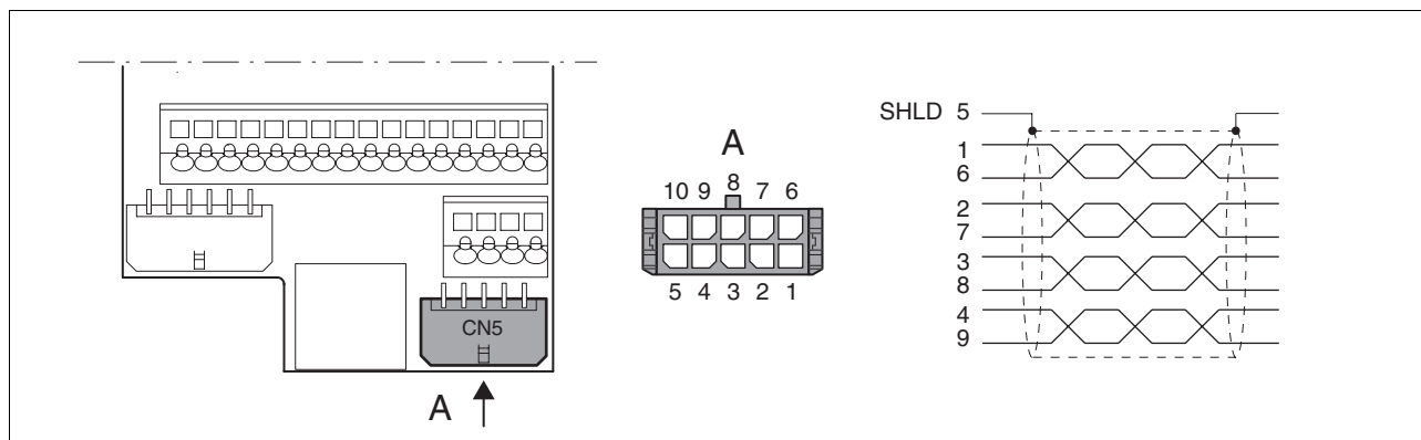
Bild 3.1 Anschlussbild CN5
