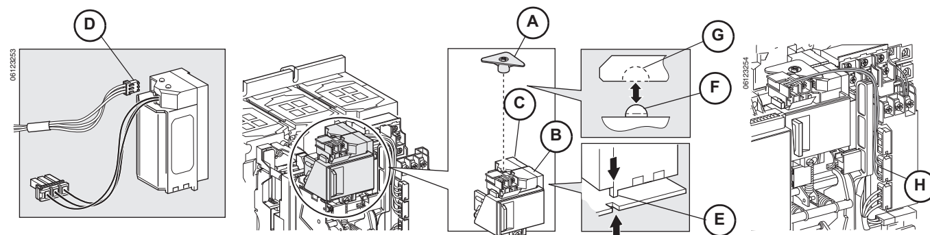
Figure / Figura / Figure 3 : Coil Replacement / Sustitución de la bobina / Remplacement de la bobine
