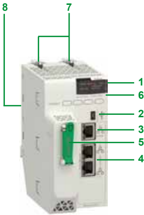
BMEP58●●●●
