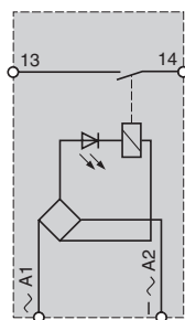
ABR2●B312B (≍ 24 V)
