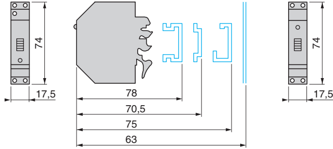
ABR 1S
