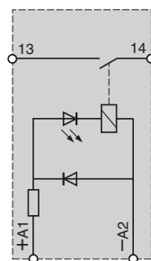
ABR2S112B (≍ 24 V)
