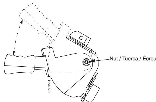
Figure / Figura / Figure 4 : Switch Handle Movement / Movimiento de la palanca del interruptor / Mouvement de la manette de l'interrupteur
