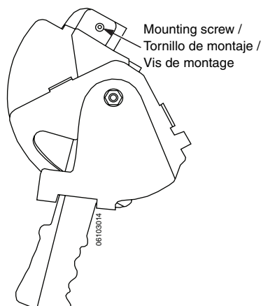
Figure / Figura / Figure 2 : Switch Handle in OFF (O) Position / Palanca del interruptor en la posición de abierto (O) / Manette de l'interrupteur sur la position d'arrêt (O)
