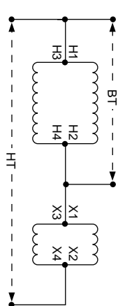
Schéma de câblage 1
