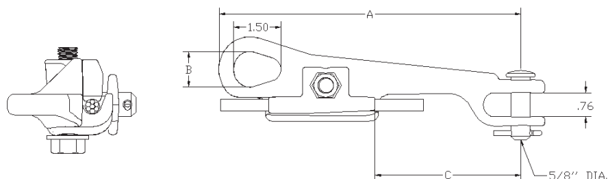
SOCKET TYPE SA
