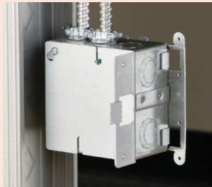
4" stud depth
