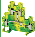
NSYTRV44DPE
