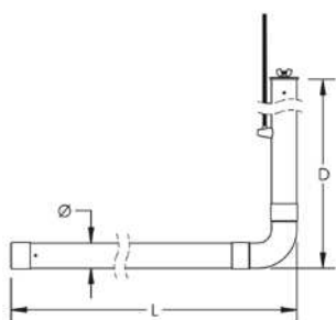
Horizontal mit beweglicher Anschlussleitung nach oben
