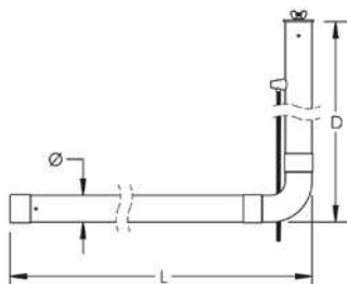
Horizontal mit beweglicher Anschlussleitung nach unten
