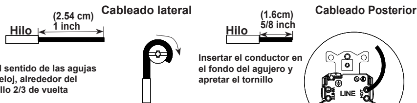
Conexiones de los conductores
