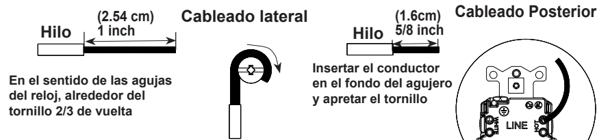
Conexiones de los conductores
