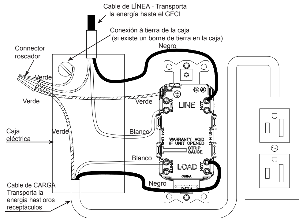
Conexiones de los conductores
