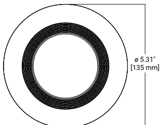
LT4 - Baffle
