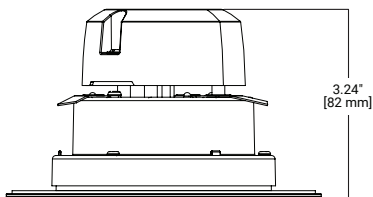
LT4 - Baffle
