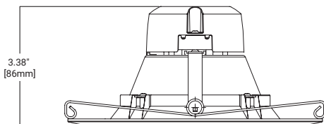
LT56 - Baffle
