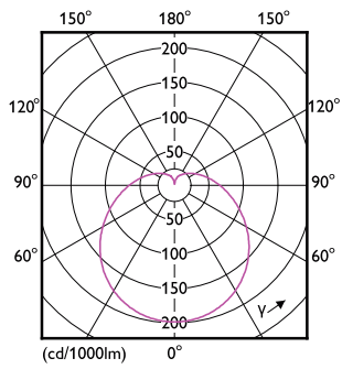
Light Distribution Diagram - 8.5A19/LED/827/FR/P/ND 4/2FB
