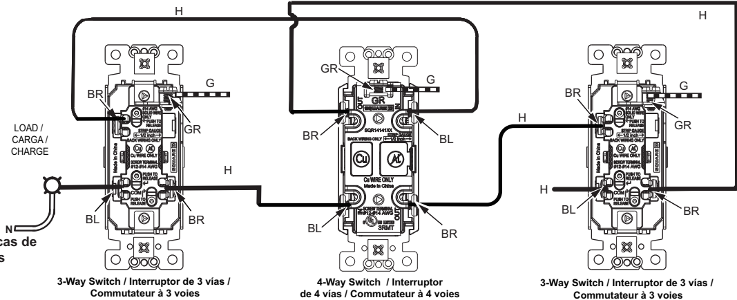
FIG 3: Wiring Diagram for SQR14141XX / SQR14231XX / Diagrama de cableado / Schéma de câblage
