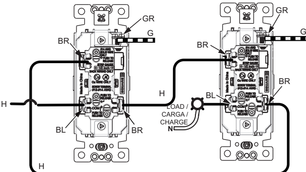
FIG 3: Wiring Diagram for SQR14141XX / SQR14231XX / Diagrama de cableado / Schéma de câblage
