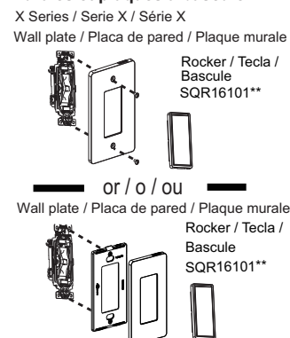
FIG 4: Wall Plates and Rockers / Placas de pared y placas basculantes / Plaques murales et plaques à bascule
