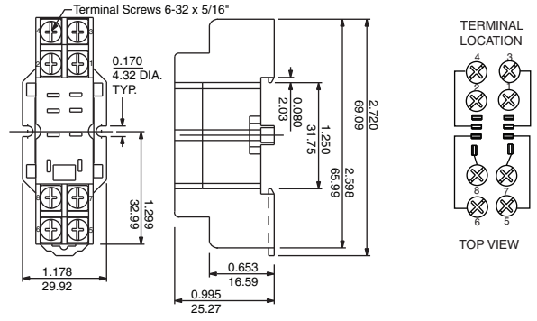
Type NR42
