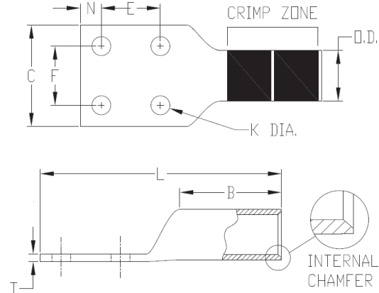
YAB-4N
