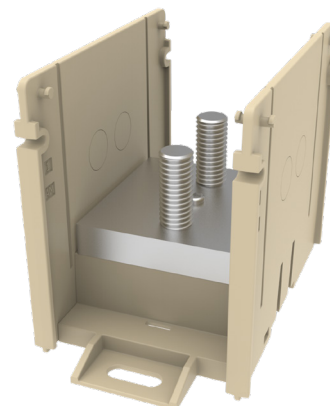
Stud-to-Stud BDBLCS5SA1 shown
