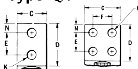
Type QA
