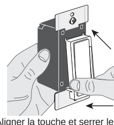
Aligner la touche et serrer les languettes latérales
