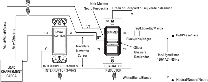
FIGURA 2: DIAGRAMA DE CABLEADO DE 3-VÍAS
