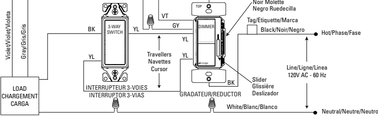
FIGURA 2: DIAGRAMA DE CABLEADO DE 3-VÍAS
