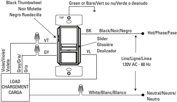
FIGURA 1: DIAGRAMA DE CABLEADO UNIPOLAR
