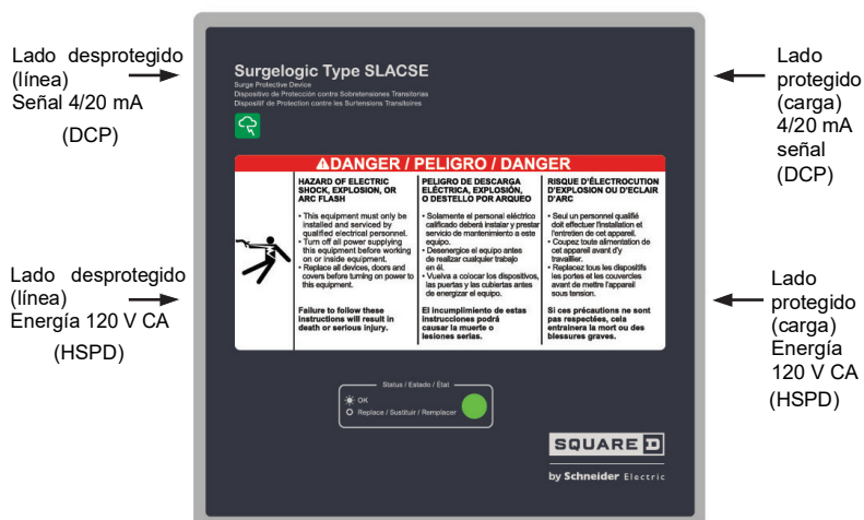
Figura 2: Instalación tipo SLACSE
