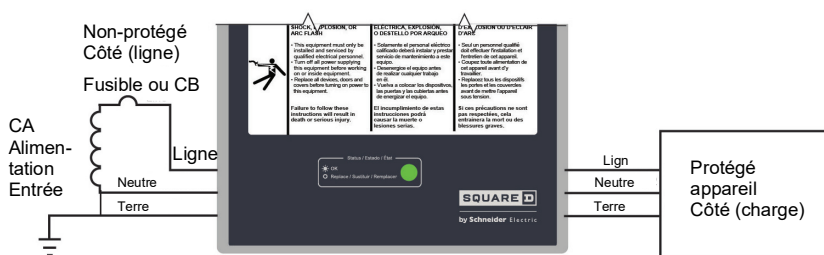
Figure 3 : Schéma de câblage du Type SLACSE
