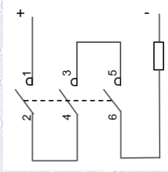
3P 外形三极串 (LC1G250DC)
