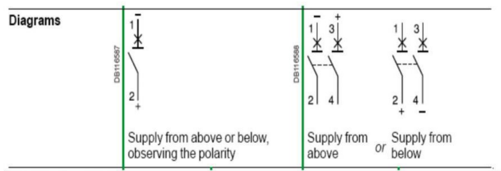
直流接线图
