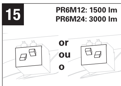
One switch up / one switch down Un interrupteur remonté/un interrupteur abaissén Un interruptor arriba / un interruptor abajo
