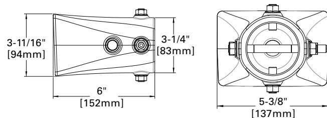
ADJA=Adjustable Pole Mount Arm (USSL-M)
