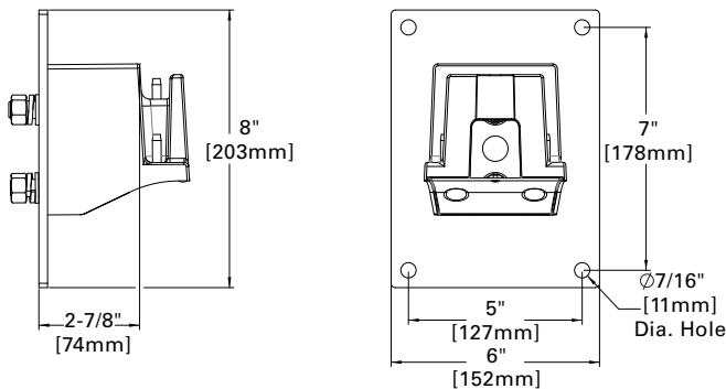
MA=QM Mast Arm (USSL-M)
