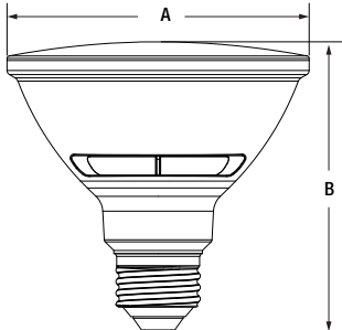
PAR30
