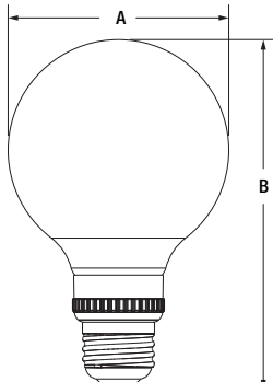
G25
