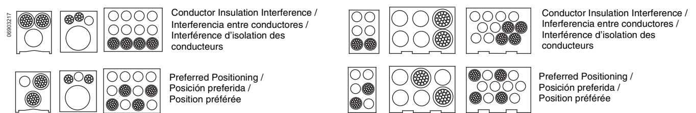
Figure / Figura / Figure 1 : Conductor Positioning / Posición de los conductores / Emplacement des conducteurs
