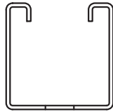
Auslegerkonsole Schienenhöhe 21 mm, Langloch
